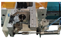
稳定可靠的动刀剪线系统
